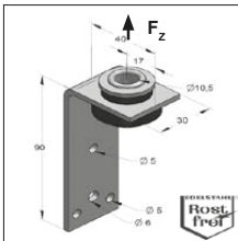
Uchwyt LLN
