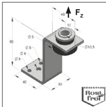
Uchwyt ZLN
